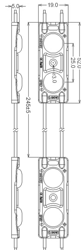
Abbildung 2: Moduldimensionen
